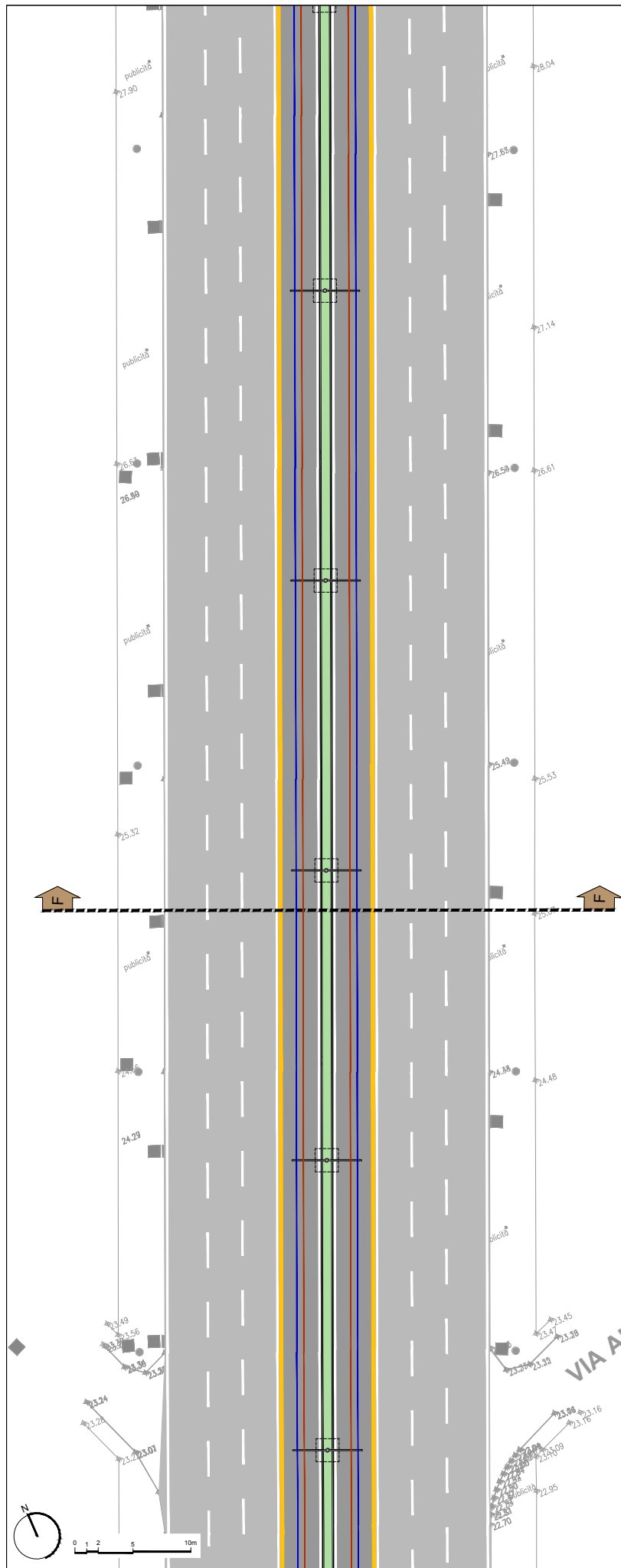
PLANIMETRIA scala 1:500
